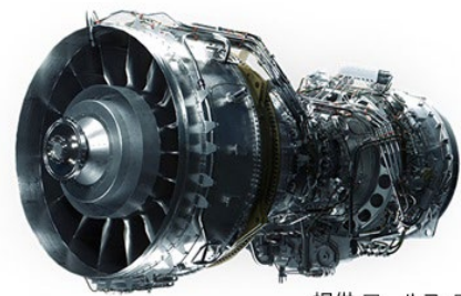
MT30 型エンジン
